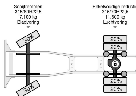
Renault Magnum 440 E-TECH (EURO 3 / ZF16 MANUA... 4x2
