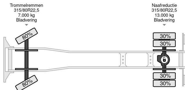
Mercedes-Benz SK 1635K 4x2 FULL STEEL MEILLER KIPP...
